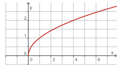
y = \sqrt{x}
