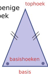
gelijkzijdige driehoek
